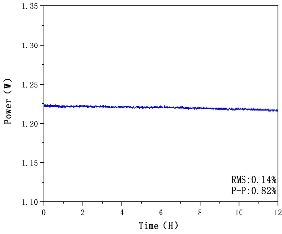
功率稳定性测试
