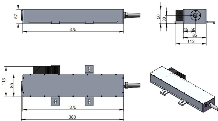
单通级联倍频输出腔尺寸图
