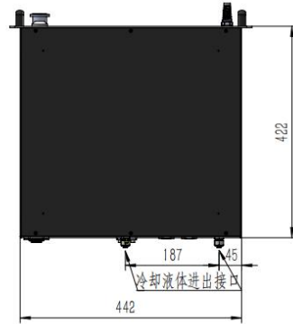
机箱尺寸图-水冷
