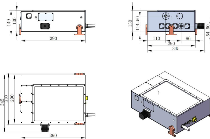
输出腔尺寸图
