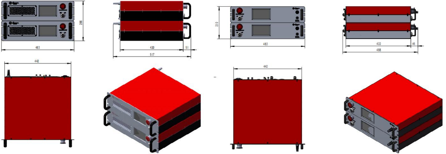
双机箱尺寸图-风冷
